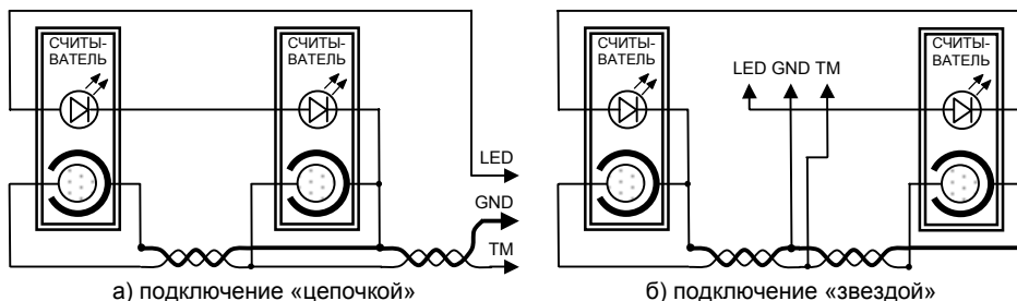
Рисунок 10 – Подключение двух считывателей
