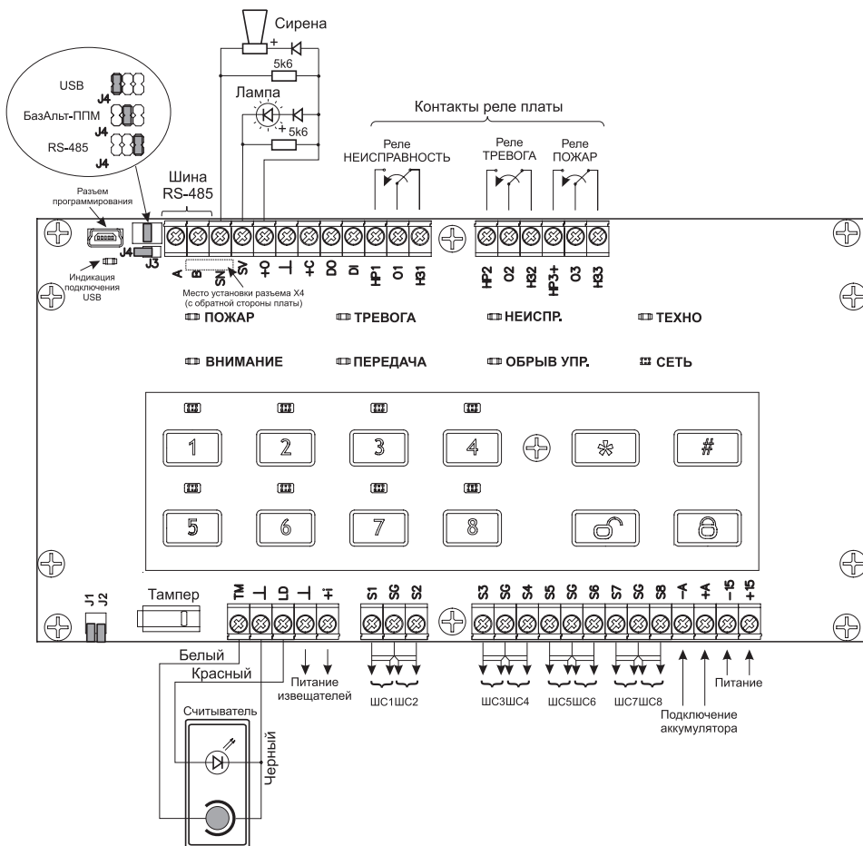
Рисунок 12 – Монтажная схема охранной панели прибора
