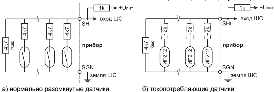
Рисунок 9 – Примеры монтажа пожарных двухпороговых шлейфов
