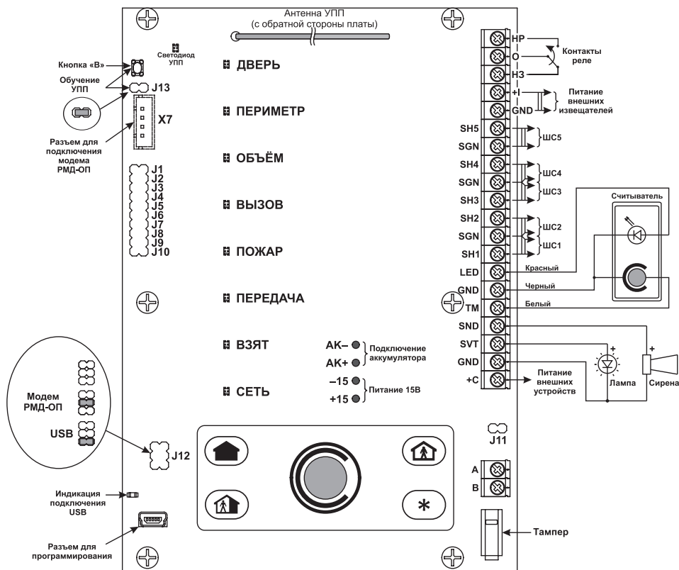
Рисунок 9 – Монтажная схема прибора
