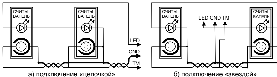
Рисунок 5 – Подключение двух считывателей
