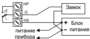
б) подключение замка, отпирающегося снятием питания
