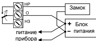
а) подключение замка, отпирающегося подачей питания
