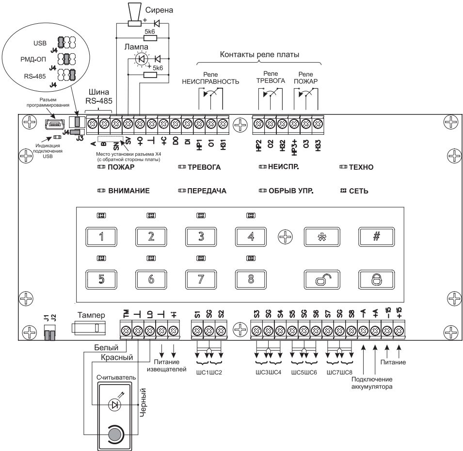
Рисунок 10 – Монтажная схема прибора
