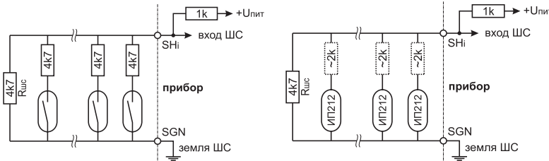
а) нормально разомкнутые датчики
