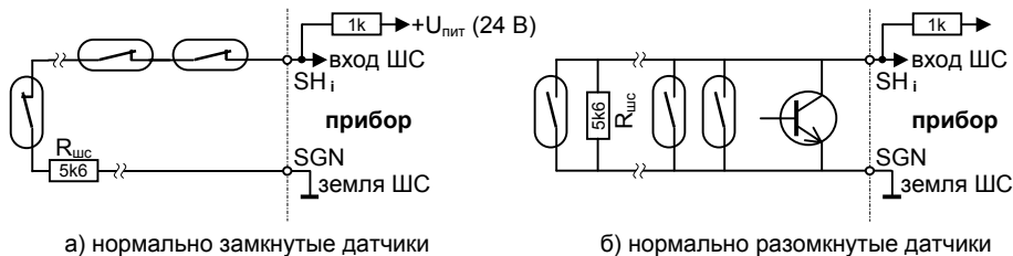
Рисунок 6 – Примеры монтажа охранных шлейфов
