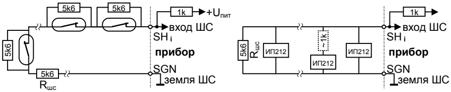
а) нормально замкнутые датчики
