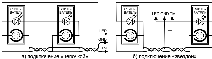
Рисунок 9 – Подключение двух считывателей
