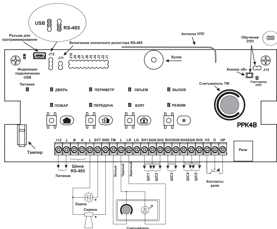
Рисунок 8 – Монтажная схема прибора
