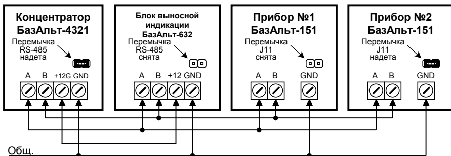
Рисунок 1 – Пример подключения приборов к концентратору
