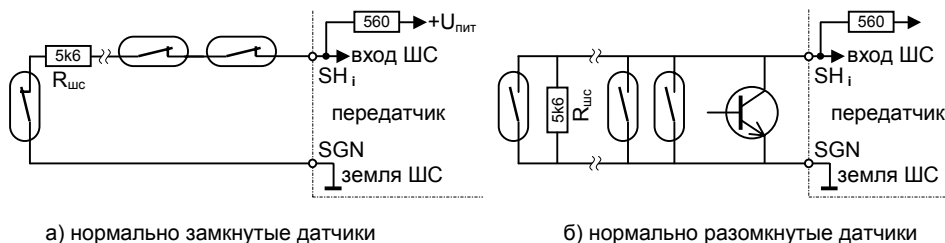
Рисунок 4 – Примеры монтажа шлейфов сигнализации
