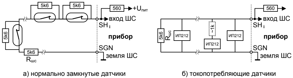
Рисунок 5 – Примеры монтажа пожарных шлейфов
