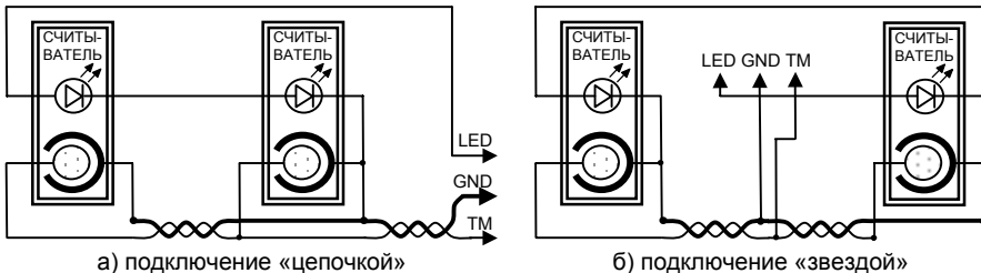
Рисунок 6 – Подключение двух считывателей
