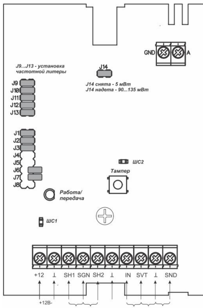
Рис. 6б. Монтажная схема RS-202TF-RR
