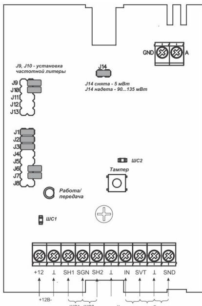
Рис. 6а. Монтажная схема RS-201TF-RR
