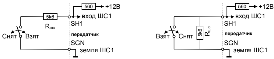
Рис. 4. Примеры монтажа ШС1 в качестве входа постановки/снятия с охраны
