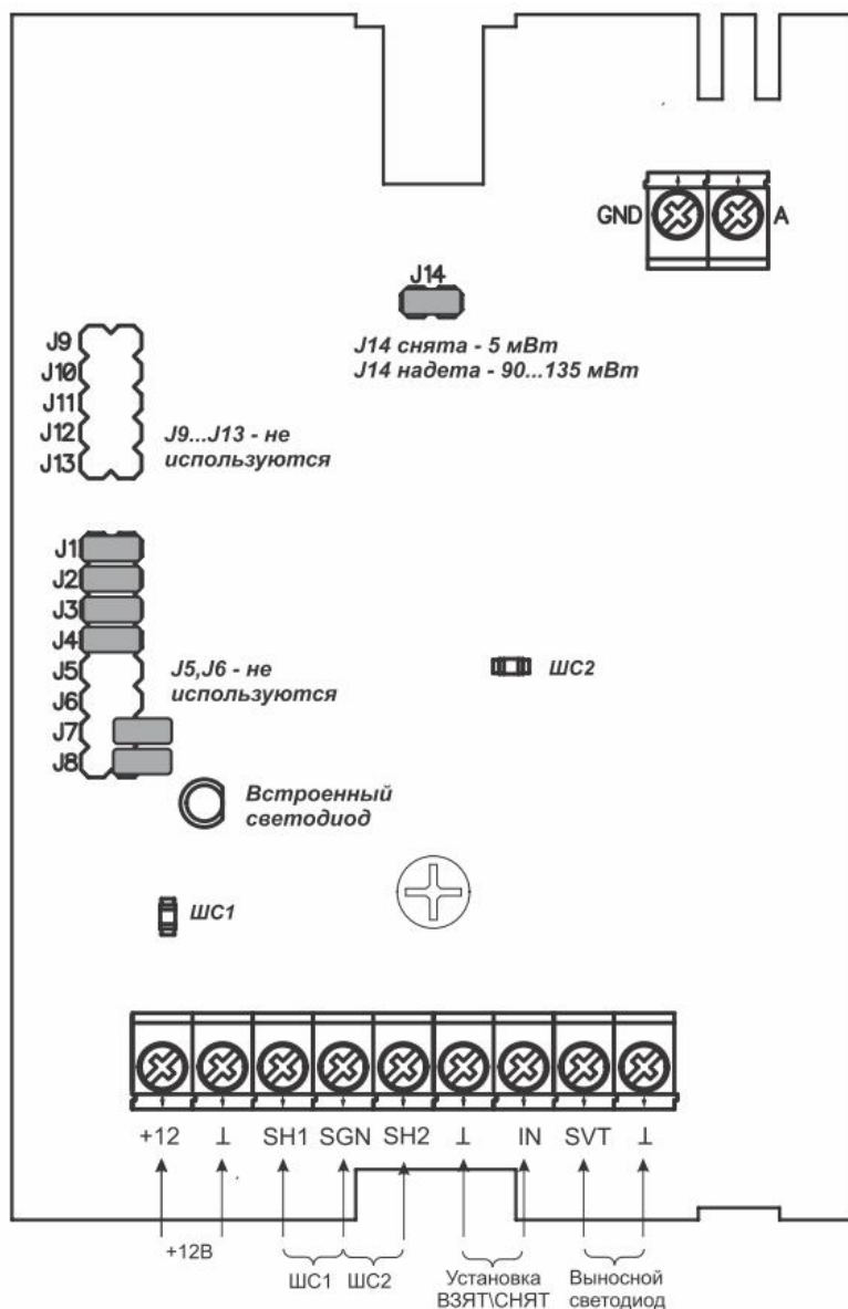
Рис. 2. Монтажная схема RR-701TS-L
