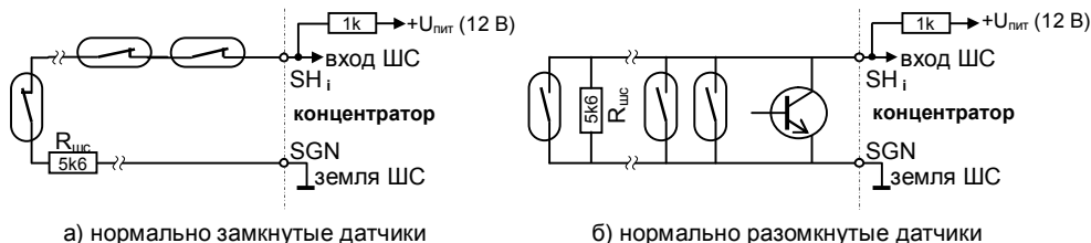
Рис. 5 – Примеры монтажа охранных шлейфов
