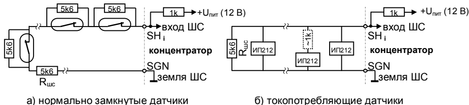
Рис. 6 – Примеры монтажа пожарных шлейфов
