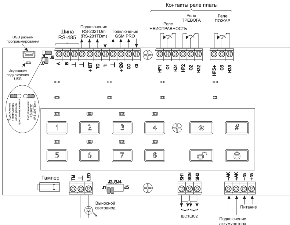
Рис. 8 – Монтажная схема концентратора
