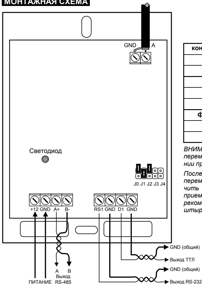
Рис. 2. Монтажная схема приемника
