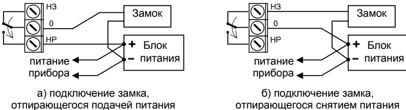
Рис. 12. Подключение электрического замка
