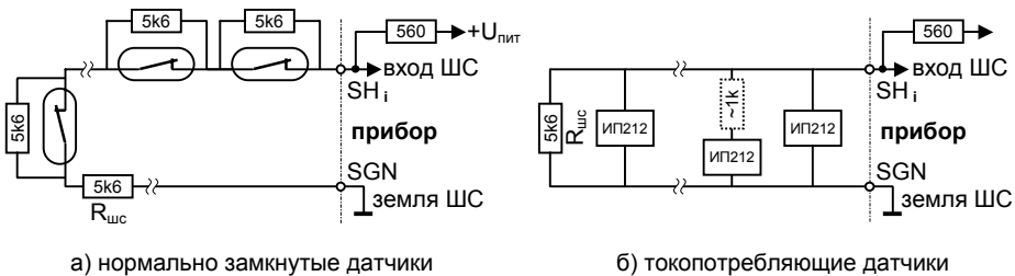
Рис. 10. Примеры монтажа пожарных шлейфов
