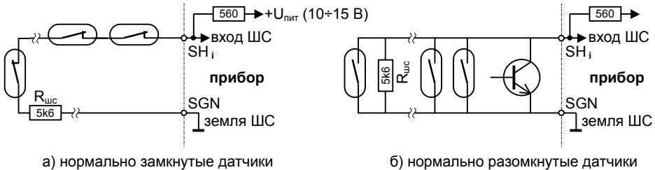
Рис. 9. Примеры монтажа охранных шлейфов
