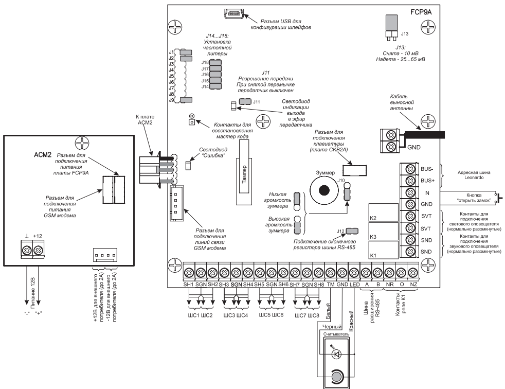
Рис. 14. Монтажная схема прибора
