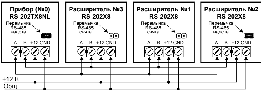
Рис. 13. Пример подключения расширителей к прибору.
