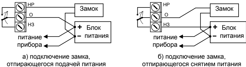
Рисунок 10 – Подключение электрического замка
