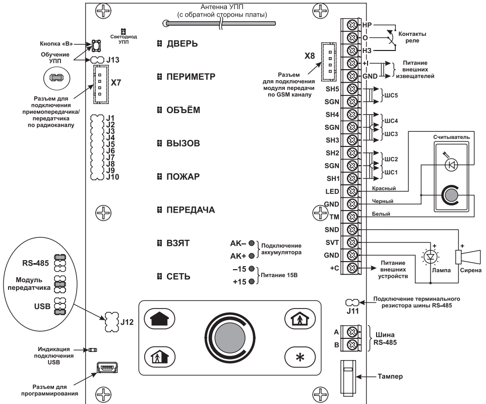
Рисунок 11 – Монтажная схема прибора
