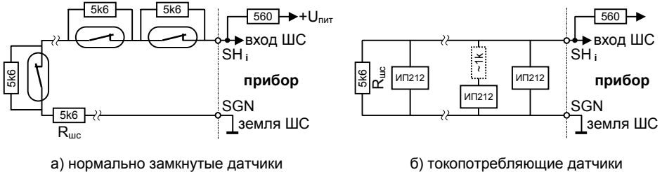
Рисунок 8 – Примеры монтажа пожарных шлейфов
