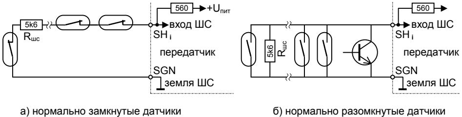
Рисунок 7 – Примеры монтажа шлейфов сигнализации
