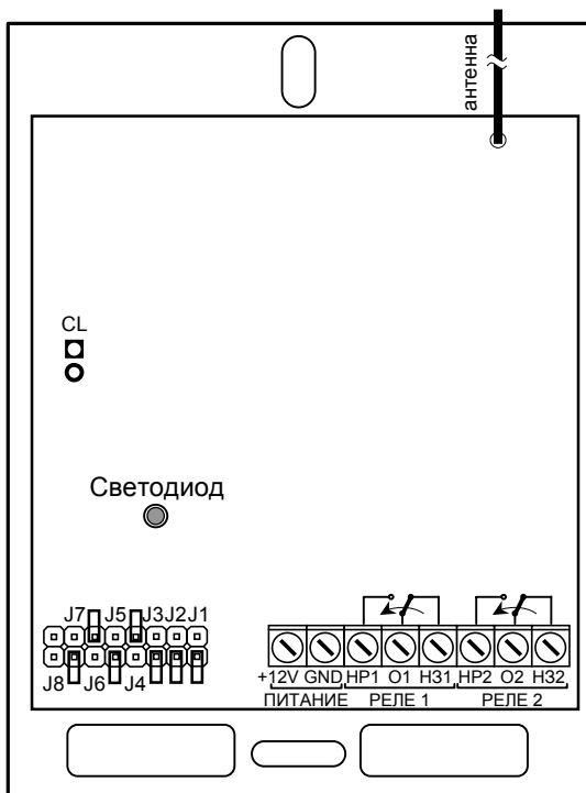
Рис. 2. Монтажная схема приемника
