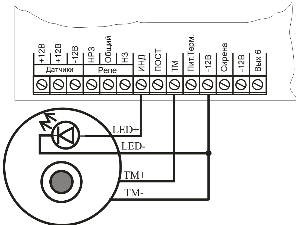
Клемная колодка Часовой 8x8-BOX
