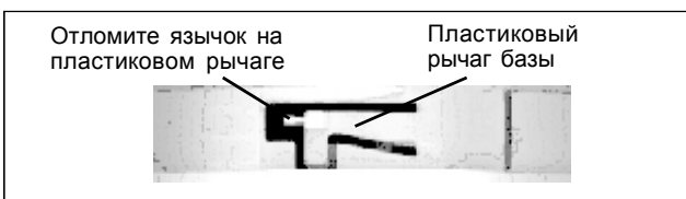
Рис. 3. Активизация функции защиты от несанкционированного извлечения извещателя
