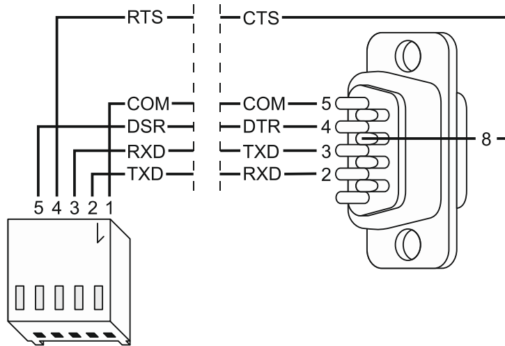
Рис. 5. Подключение ПК к последовательному порту АСУ-100. С левой стороны вид разъема PIN5. С правой – разъем типа «мама» DB-9 со стороны точек пайки.
