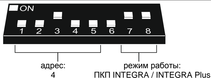
Рис. 7. Пример установки DIP-переключателей.
