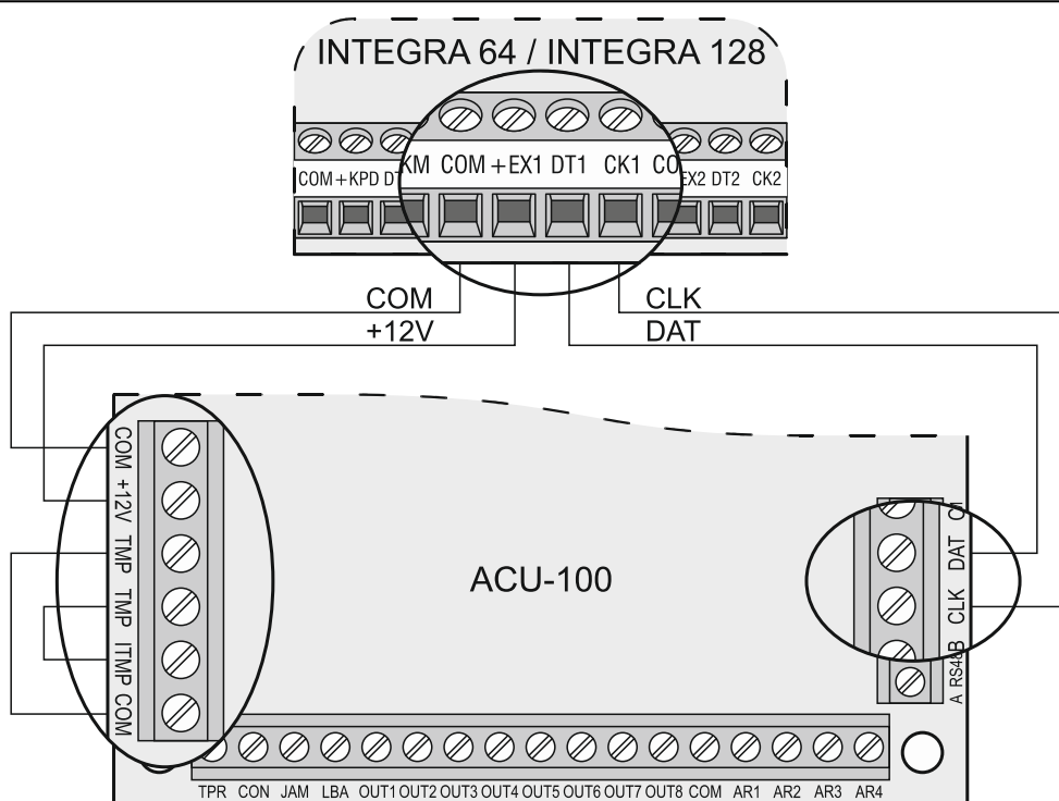
Рис. 8. Пример подключения контроллера ACU-100 к ПКП INTEGRA.
