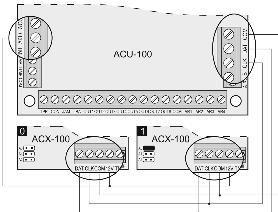
Рис. 6. Пример подключения 2 модулей АСХ-100 (адреса: 0 и 1) к контроллеру АСУ-100.
