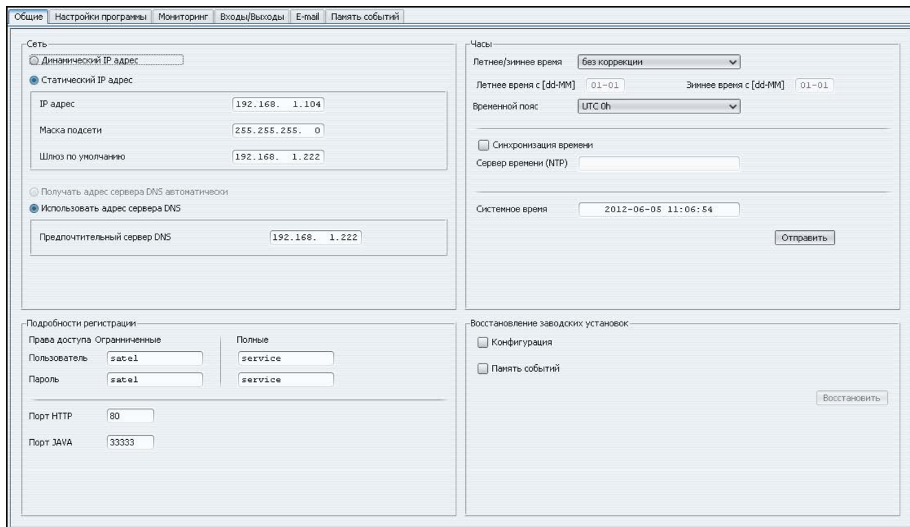
Рис. 4. Вкладка «Общие».
