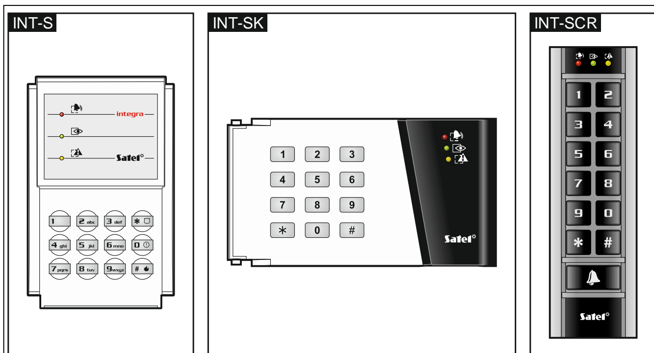
Рис. 4. Групповые клавиатуры (клавиатуры INT-S и INT-SK, представленные без откидной крышки).
